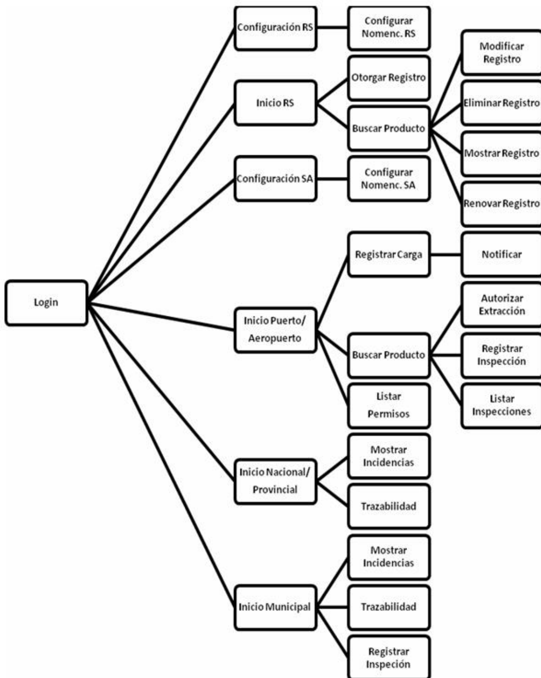
Fig. 2. Mapa de navegación del Módulo Salud Ambiental.
