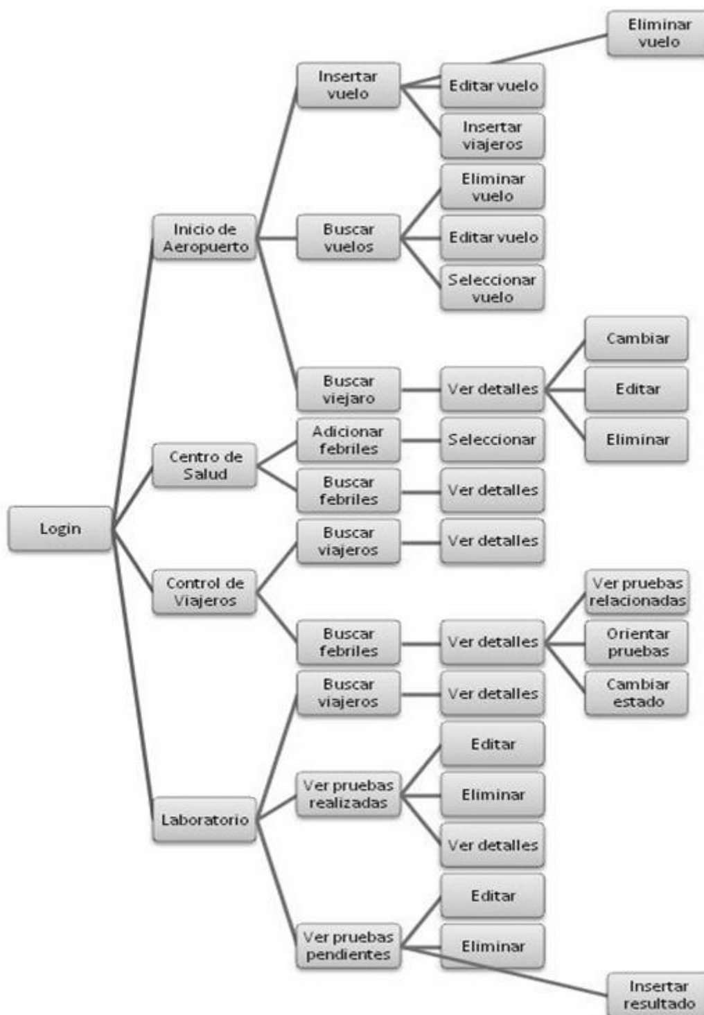
Fig. 3. Mapa de navegación del Módulo Higiene y Epidemiología.
